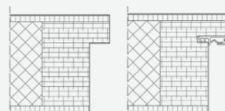
Standard tiefler Einfachfalz
