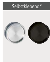
Griffmuschel Amrum für Glastüren, Edelstahlfarbig und Schwarz Aussenmasse: Ø 50 u. 65 mm
