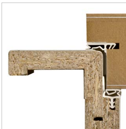
Zwei Dichtungsebenen durch die integrierte Türfalzdichtung und die akustisch wirksame Zargendichtung.
