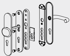
Schutzbeschlag ES 1
