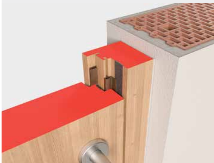
EI 60 Pfostenstock flächenbündig mit Aufdoppelung
