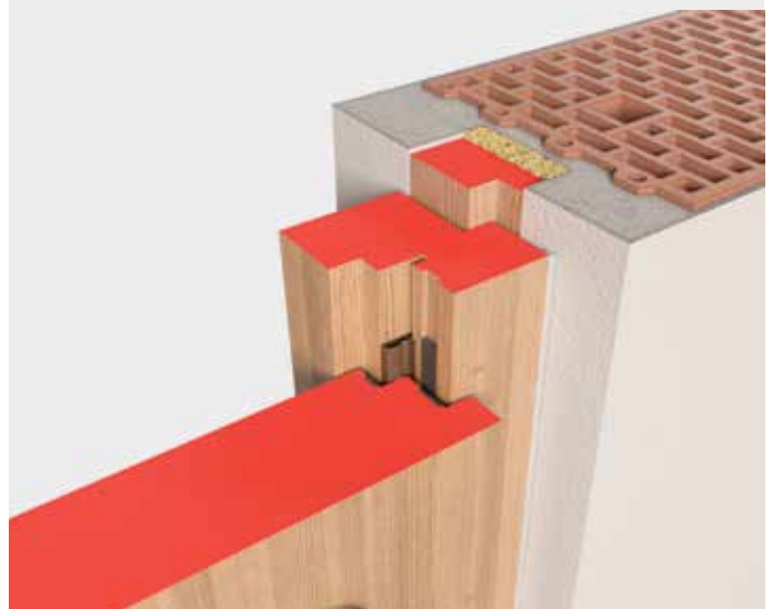
EI 60 Pfostenstock überfäلت (Optional Schallschutztür STILL® 42 dB)
