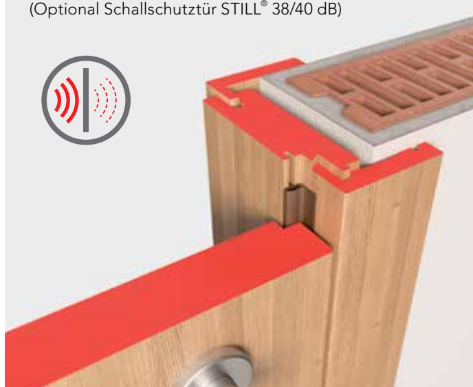
G-Zarge, flächenbündig
