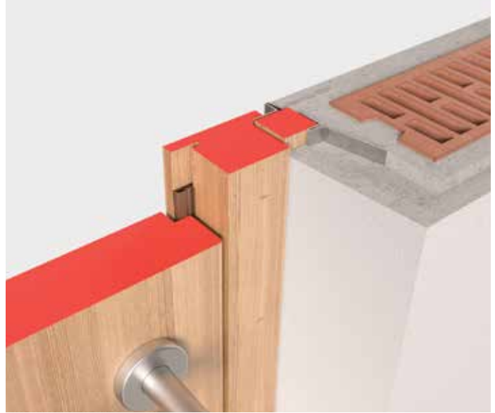
Pfostenstock M-Zarge, flächenbündig, mauerbündig
